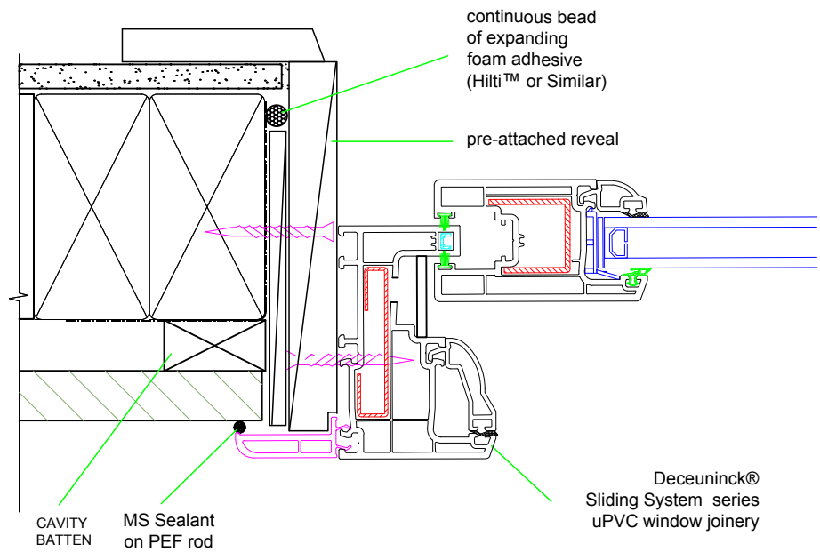
JAMB Detail CAV.WIN.R.1.J
